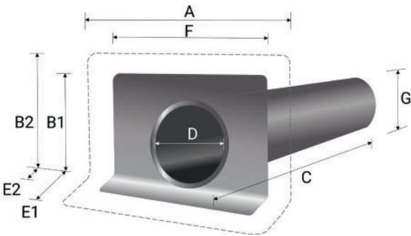
Abb. 4: Eckige Flanschausführung (PVC)
