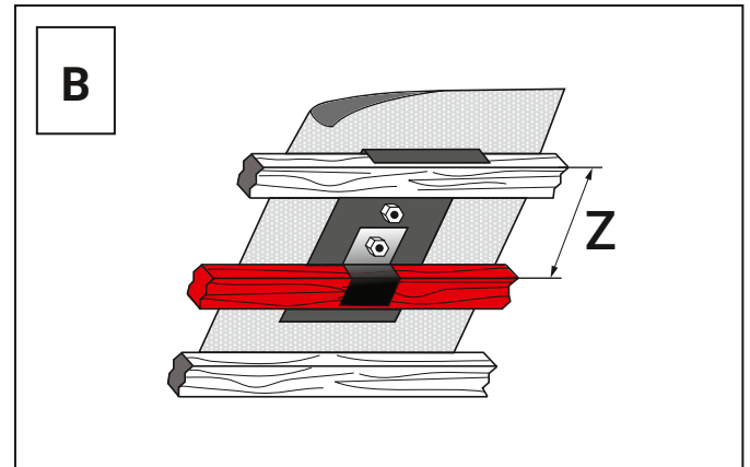
Solarflex-Universalträgerpfanne (für alle in der nachfolgenden Liste aufgeführten Pfannenmodelle mit Z = 22,5 cm einsetzbar)
