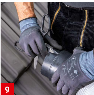
9 Rand des gekürzten Reduzierstücks mit geeignetem Werkzeug entgraten, um Einbau an die Anschlussleitung zu erleichtern 2 .
