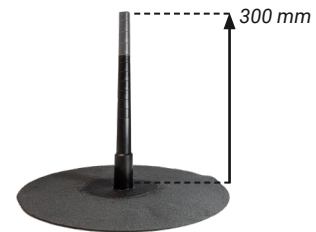
Schumpfi-XL: Zur flexiblen Einfassung von Anschlagpunkten mit Durchmessern von 22 oder 52 mm
