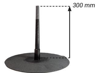
Schrumphi-XL: voor het flexibel omhullen van bevestigingspunten met een diameter van 22 of 52 mm.
