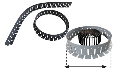
Universele grindvanger RINGO (uit één of twee delen): beschermt afvoeren zoals groendakafvoeren en de ROOFGUARD. Diameter en vorm variabel aanpasbaar aan de omstandigheden
