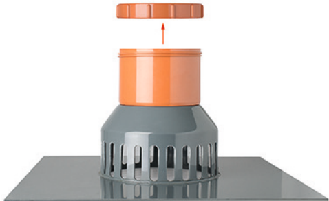
Populair op Duitse groendaken: de groendakafvoerput
