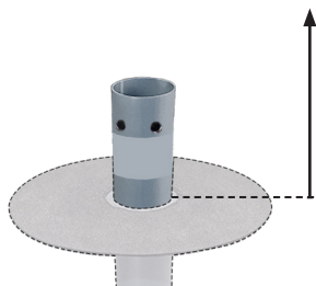
Retentieklep: wordt in de dakafvoer geplaatst en regelt zo de afwateringscapaciteit individueel. Deze is geschikt voor FLECK-afvoeren in DN 70/100/125/150.
