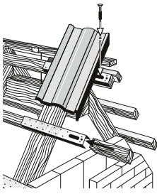
Abbildung zeigt Anbringung der Dachlattenverlängerung
