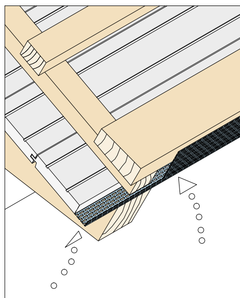
Einbaubeispiel Lüftungswinkel
