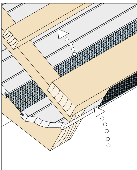
Einbaubeispiel Lüftungstreifen
